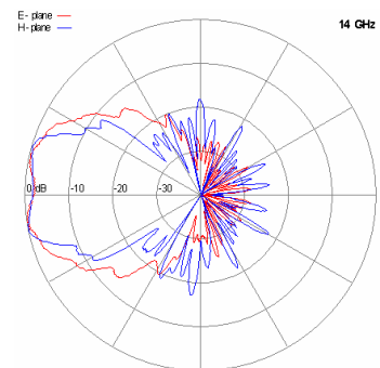
14 GHz
