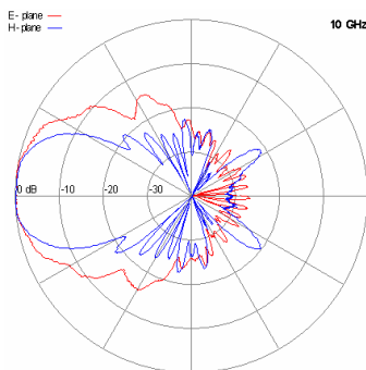
10 GHz
