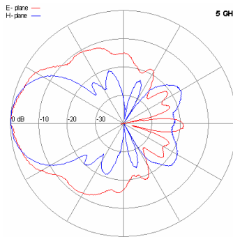
5 GHz
