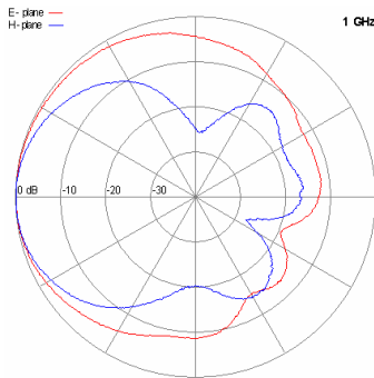
1 GHz
