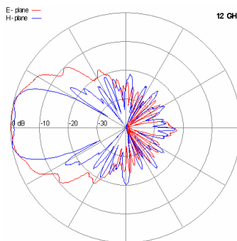
12 GHz
