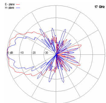
17 GHz
