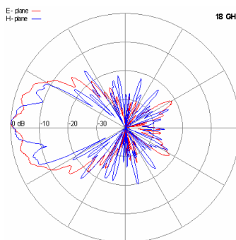
18 GHz
