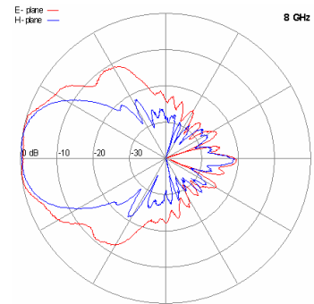
8 GHz
