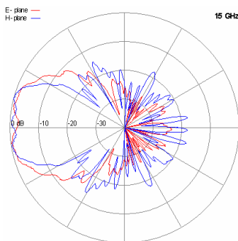
15 GHz
