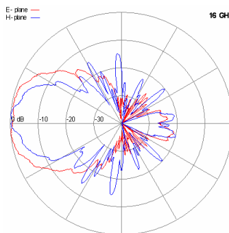
16 GHz
